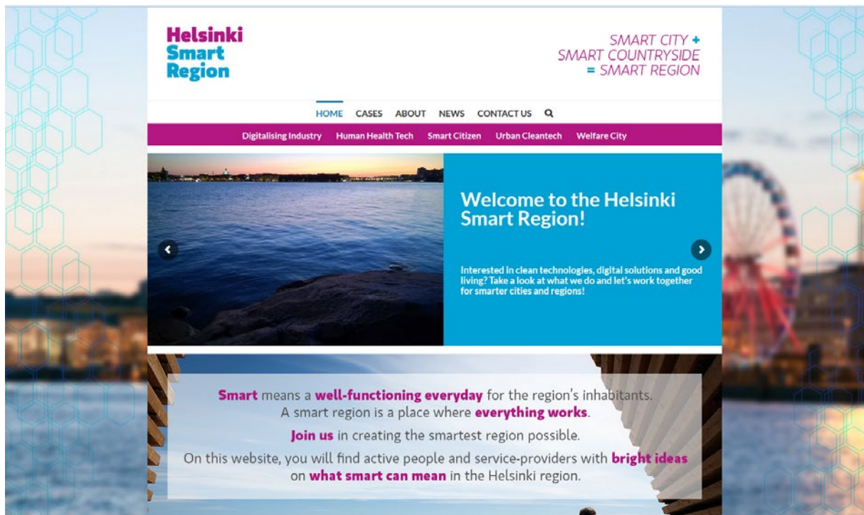
Kuva 6. Kuvakaappaus helsinkismart.fi-sivustolta.
