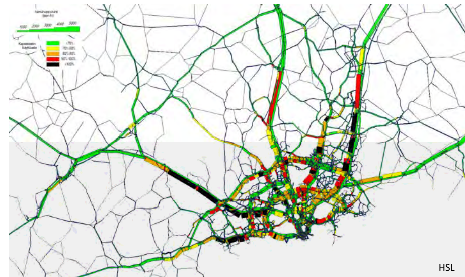
Tieverkon kuormittuminen aamuruuhkassa, H1.
