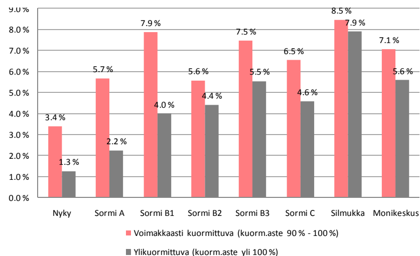
Kuva 26 Kriittisesti kuormittuvan tieverkon osuus aamuruuhkatunnin liikennesuoritteesta.
