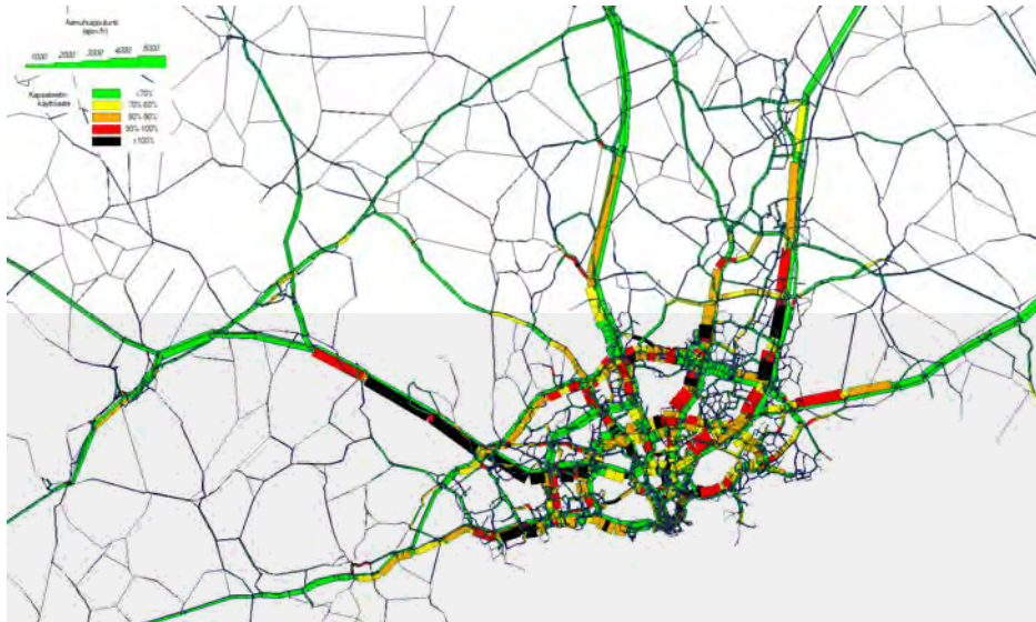
Tieverkon kuormittuminen aamuruuhkassa, H3.
