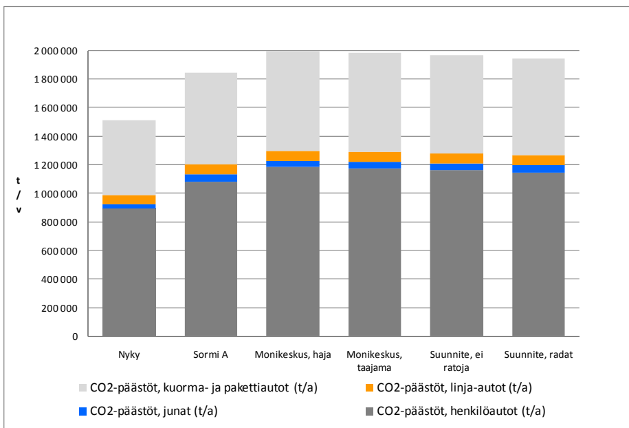
Liikenteen kasvihuonepäästöt.
